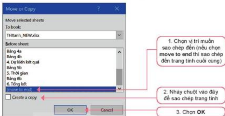
Hình 10.3. Cửa sổ Move or Copy
