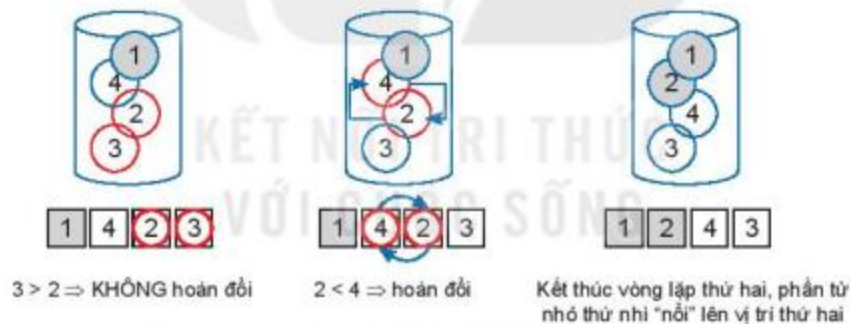
Hình 16.3. Vòng lặp thứ hai của thuật toán nổi bọt
